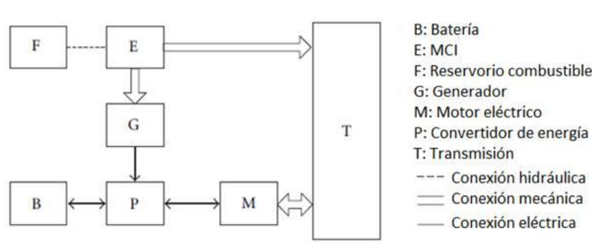
Figura 5. Configuración combinada de un HEV. Fuente: A Comprehensive Overview of Hybrid Electric Vehicles; Caiying, Peng, & Tao (2011). La siguiente tabla enlista la configuración de algunos modelos de EV.
